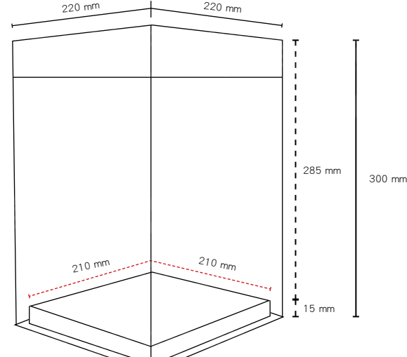
T-22 芭比 尺寸圖
