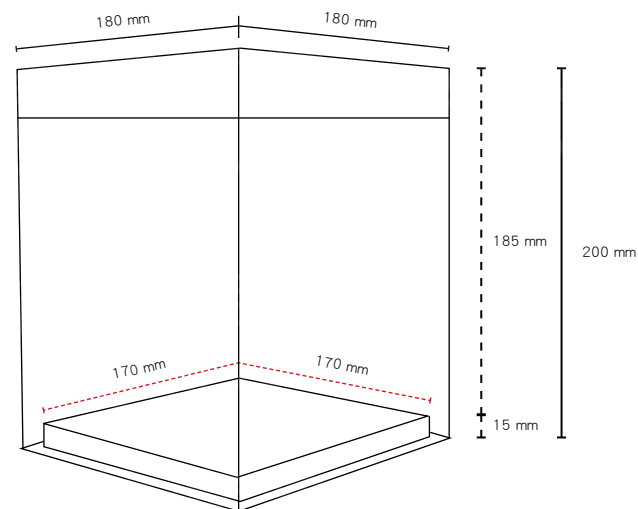
T-18 加高 尺寸圖
