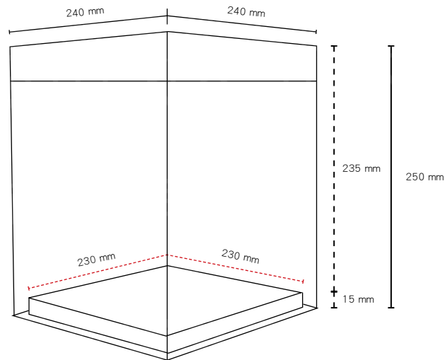
T-24 加高 尺寸圖
